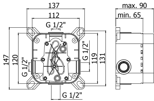
A Artt. 010-510 (senza deviatore / without diverter)
